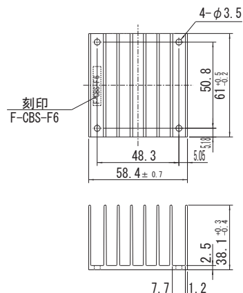
図6 F-CBS-F6の外形図
