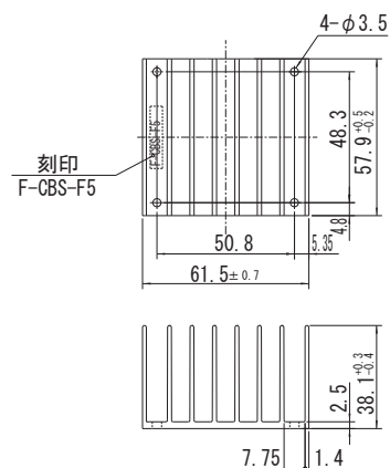
図3 F-CBS-F5の外形図
