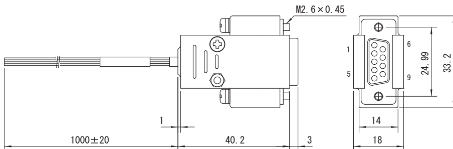
<拡張UART側>
